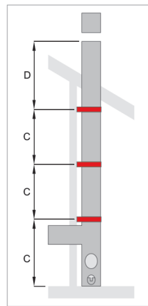
Sistema camino a vista appoggiato su di un basamento
