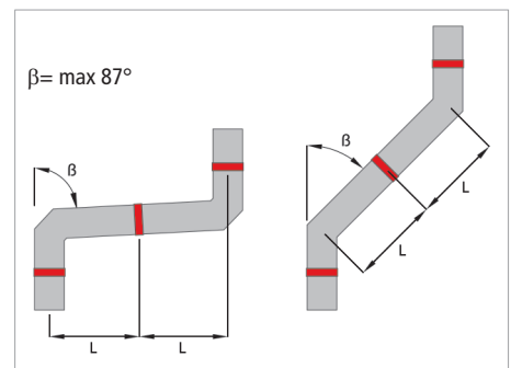
Sistema camino con spostamento
